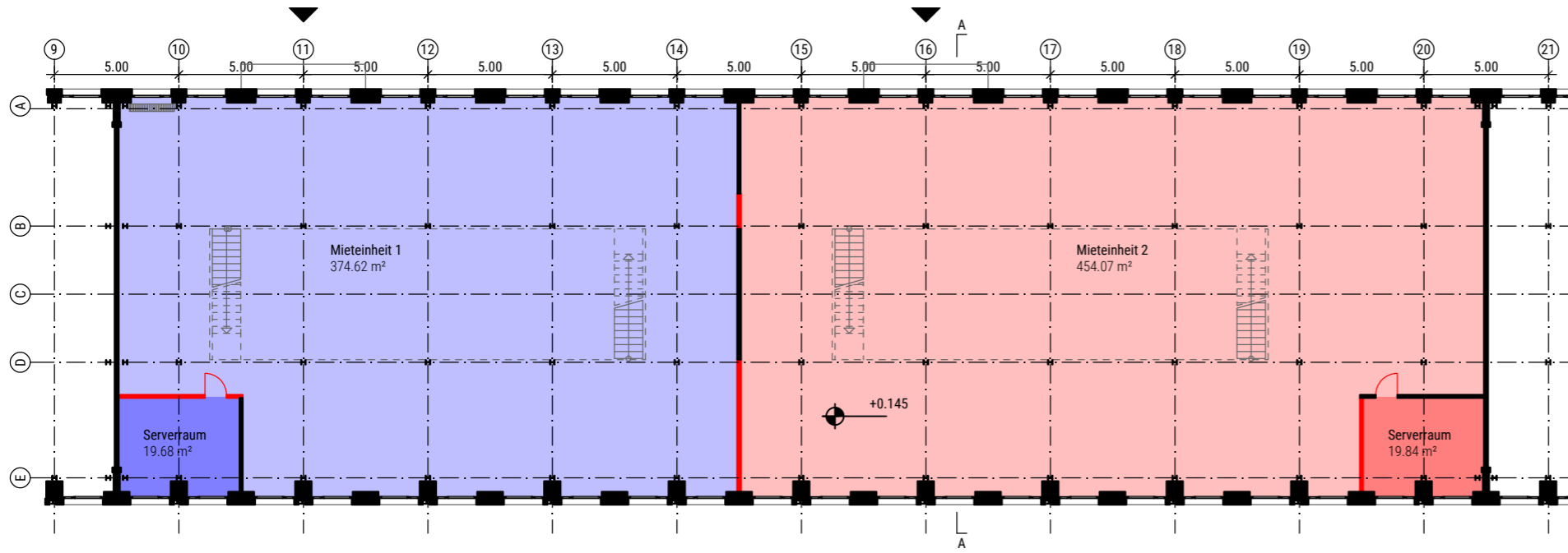
Grundriss Erdgeschoss
