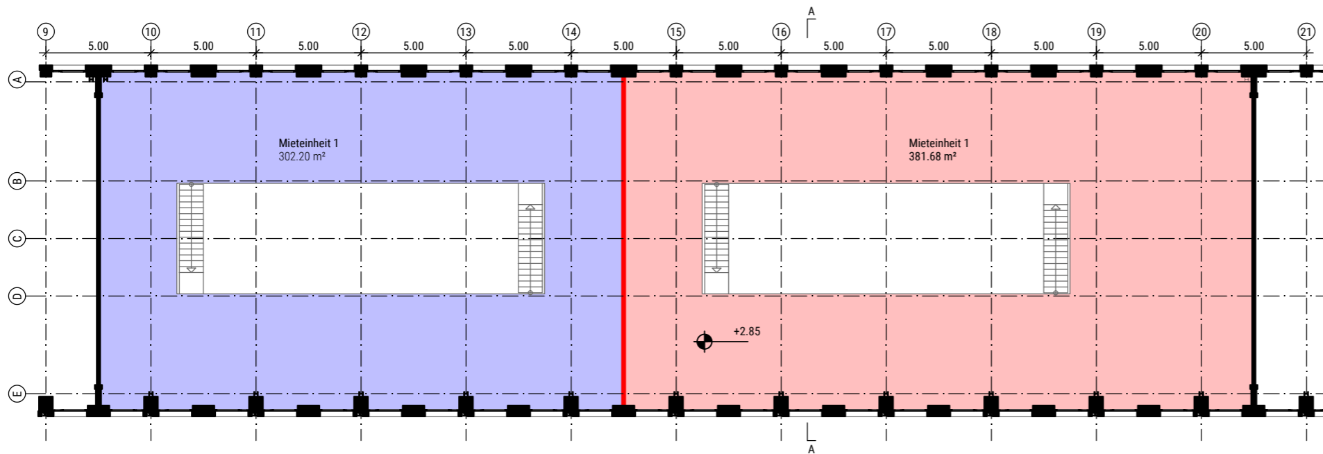
Grundriss Obergeschoss
